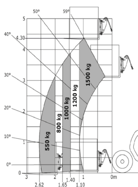
Rough terrain load chart (EN1459 B) 500 mm load center
